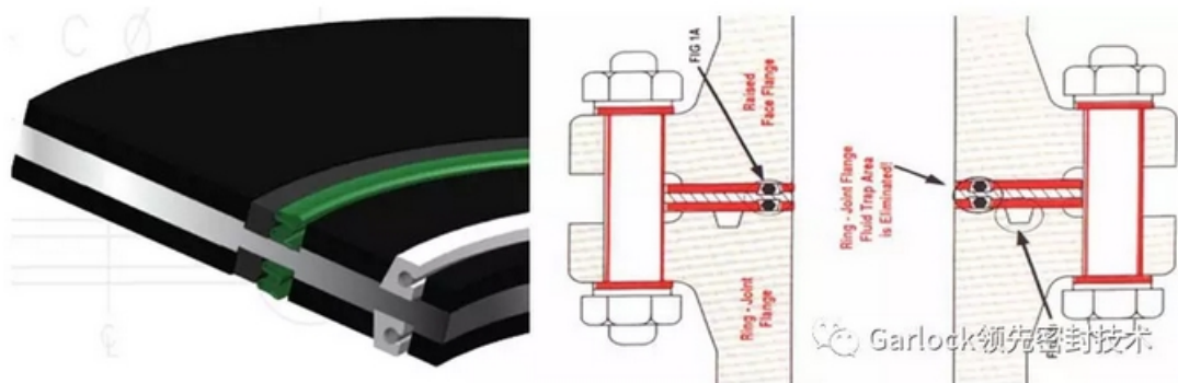
图 2: VCFS 绝缘防火型密封垫片 (剖面) 和绝缘组件的示意图
